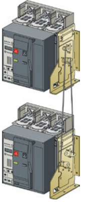
Çubuk ile dikey mekanik kilitleme
